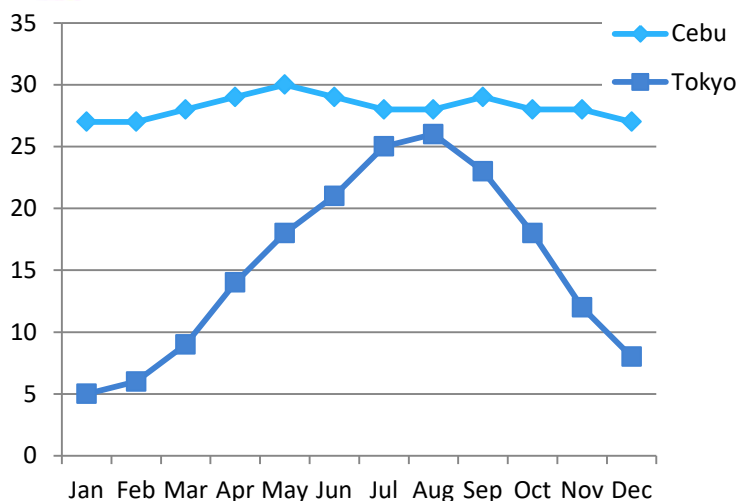
平均気温
