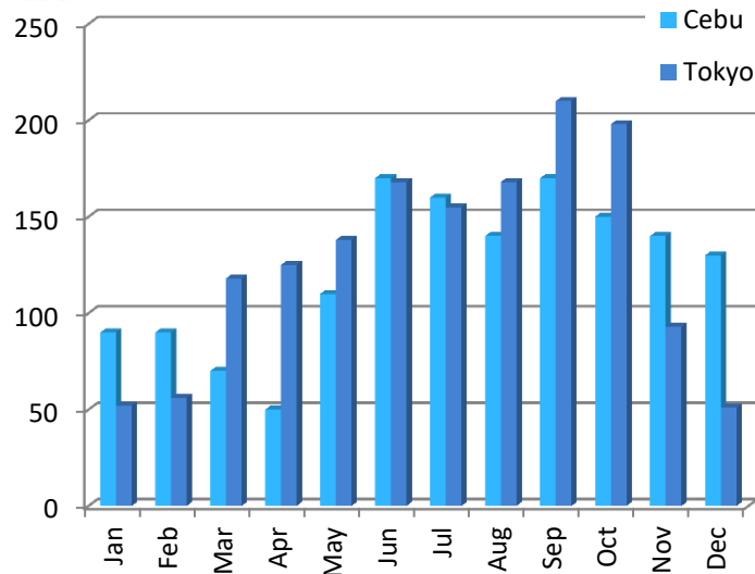
平均降水量
